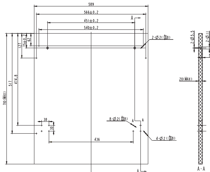
FIG. 3 Le panneau de la porte doit être placé comme décrit sur les dimensions illustrées sur ce dessin
