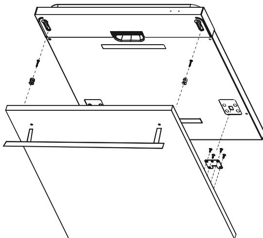
FIG 4a) Installation du panneau décoratif
